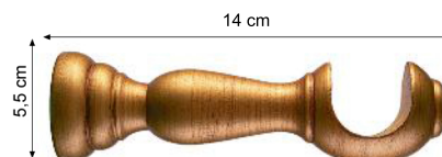
Mensola aperta Art. WD35MSA14
